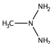
Molécule A
