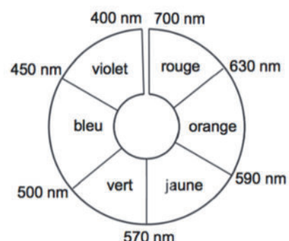
Figure 3. Cercle chromatique
